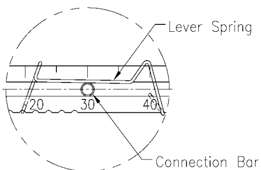
图 3-4：在杠杆和杠杆弹簧之间正确插入连接杆 (行程 30mm)
